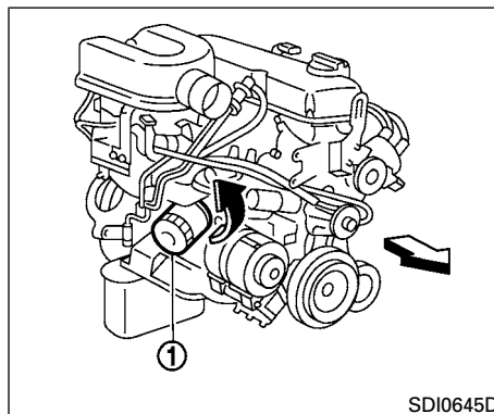
Motor KA24DE
